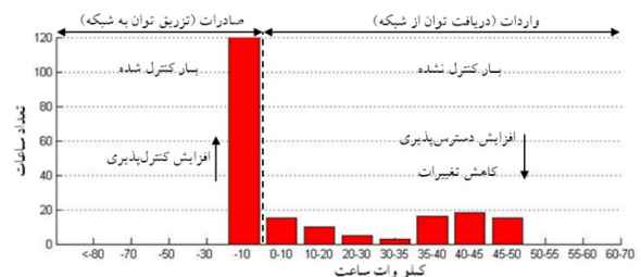
شکل (۱۱): نمودار جریان برق در PCC برای ۷ روز در روش پیشنهادی
