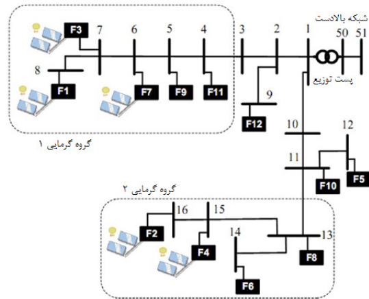
شکل (۱): سیستم ۱۸ شینه IBEE [۸]
