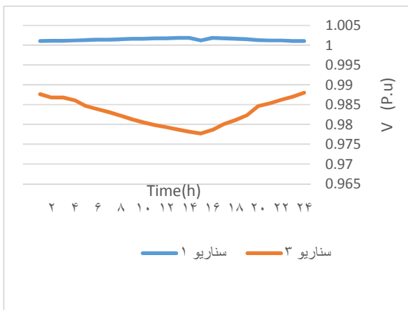
شکل (۲): پروفیل ولتاژ شین شماره ۸ در سناریوهای ۱ و ۳
