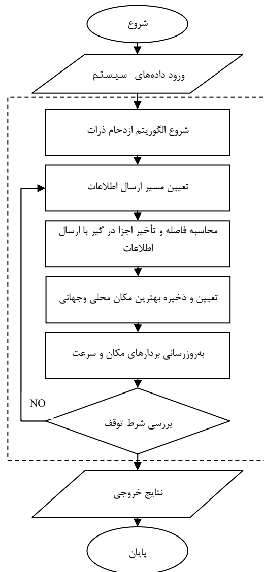
شکل (۴): روند نهایی الگوریتم بهینه‌سازی
