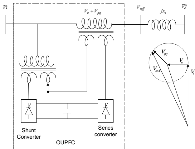
شکل ۱ دیگرام فازوری و نمای ساده یک OUPFC
