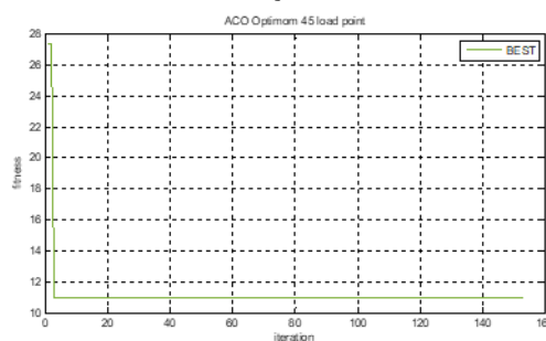
شکل (۹) : روند همگرایی الگوریتم مورچگان و الگوریتم مورچگان اصلاح شده در متعادل سازی شبکه با ۴۵ بار جدول (۳) : جریان های فاز تعادل
