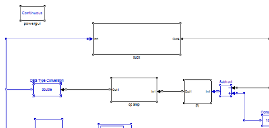
شکل ۴: شبیه سازی مبدل باک با کنترلر PI
