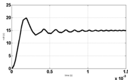
شکل ۶: موج ولتاژ خروجی مبدل باک با کنترلر SMC
