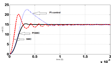
شکل ۸: موج مبدل باک با کنترلر های PI و SMC و PISMC
