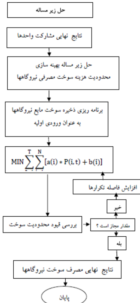
شکل (۲): الگوریتم حل زیر مسئله
