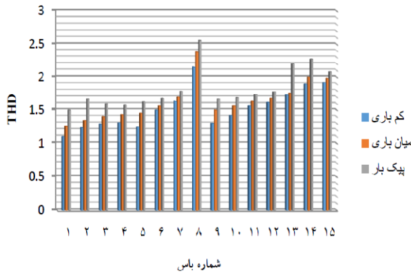
شکل (۸): پروفیل هارمونیکی شبکه ۱۵ شینه در حالت خازن‌گذاری با الگوریتم پیشنهادی (CSA)
