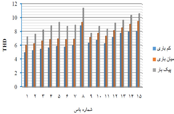
شکل (۶): پروفیل هارمونیک شبکه ۱۵ شینه در حالت بدون خازن‌گذاری
