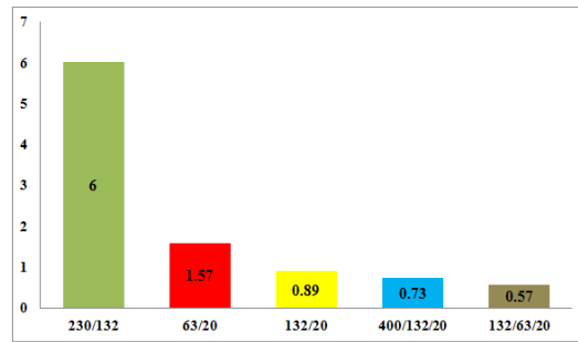
شکل ۱۳: آمار خروج ترانسفورماتورهای قدرت بر حسب تعداد حادثه به هر ترانس [۳۸]
